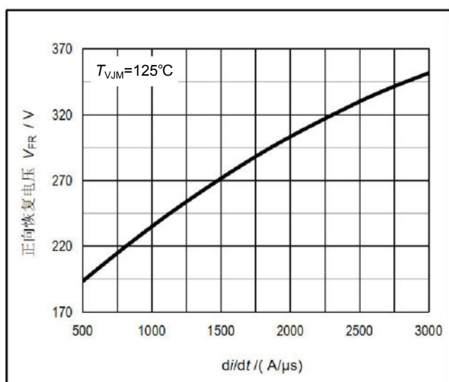
图3. 正向恢复电压与开通 di/dt 的关系曲线
