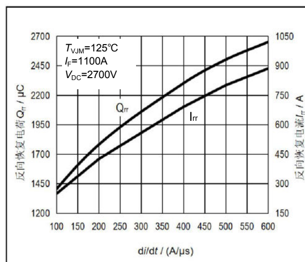
图4. 反向恢复电荷、电流与关断 di/dt 的关系曲线
